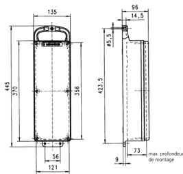
Schéma 5 MB 44
