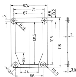
Schéma 1 MB 288 Dim. en mm
