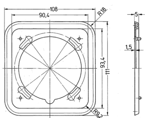
Schéma 1 MB 363 Dim. en mm
