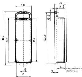
Schéma 5 MB 44 Dim. en mm
