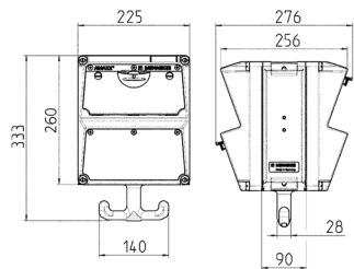
Schéma 1 MB 630
